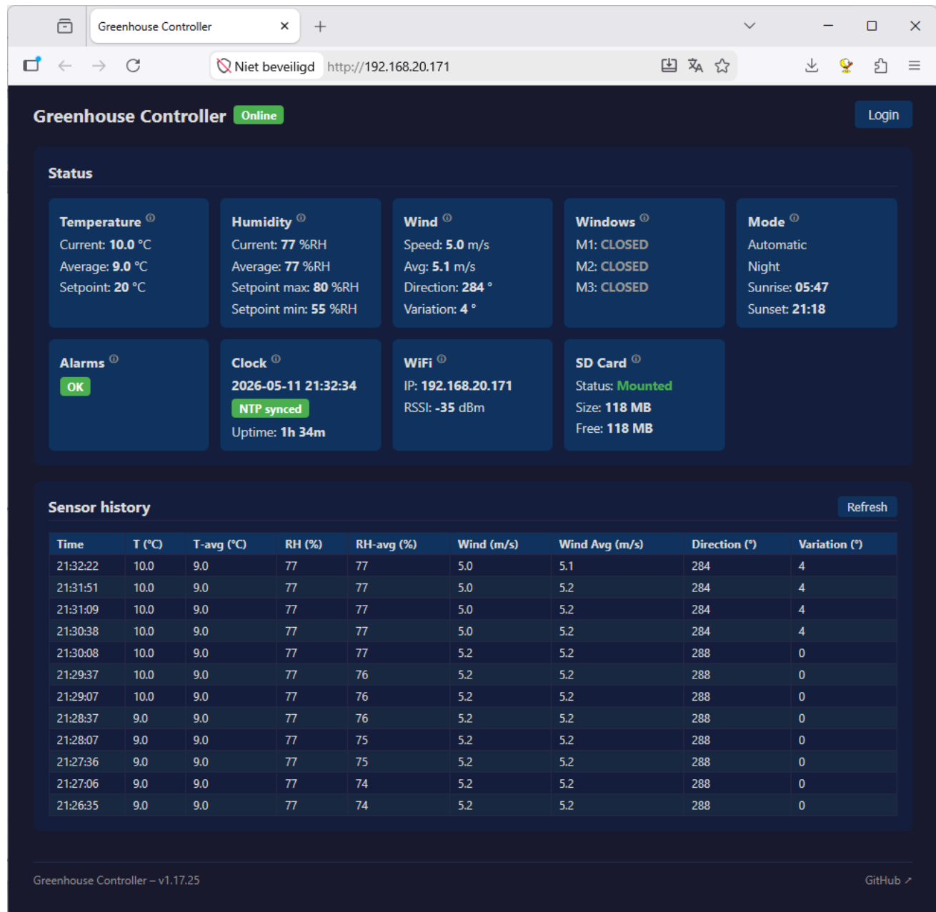
Figuur 3: hoofdpagina van de webinterface
