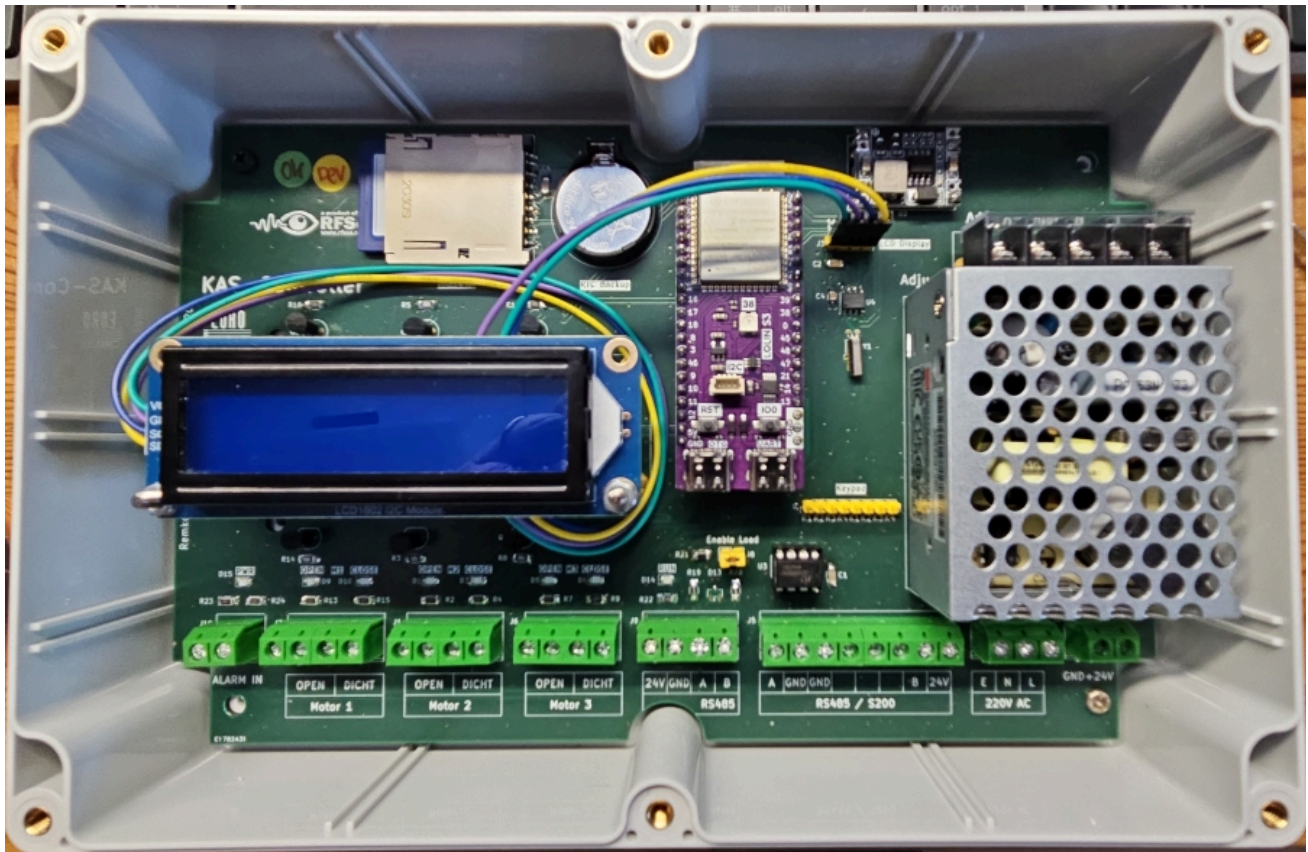
Figuur 2: Kas controller interieur.
