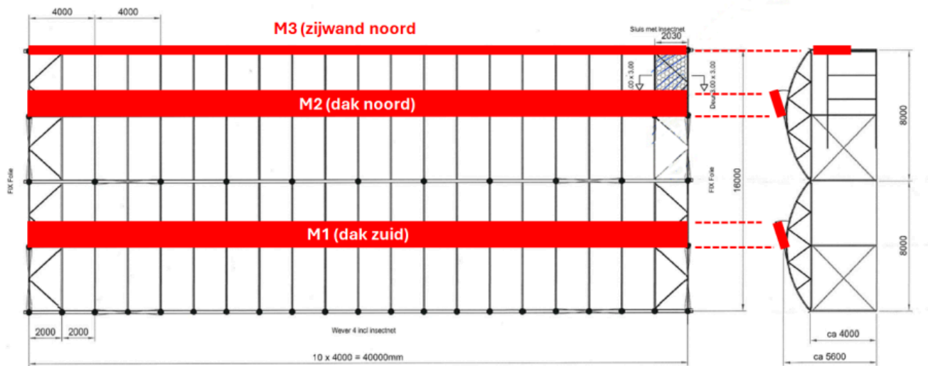
Figuur 1: bovenaanzicht / plattegrond van de kas met M1, M2 en M3 aangegeven
