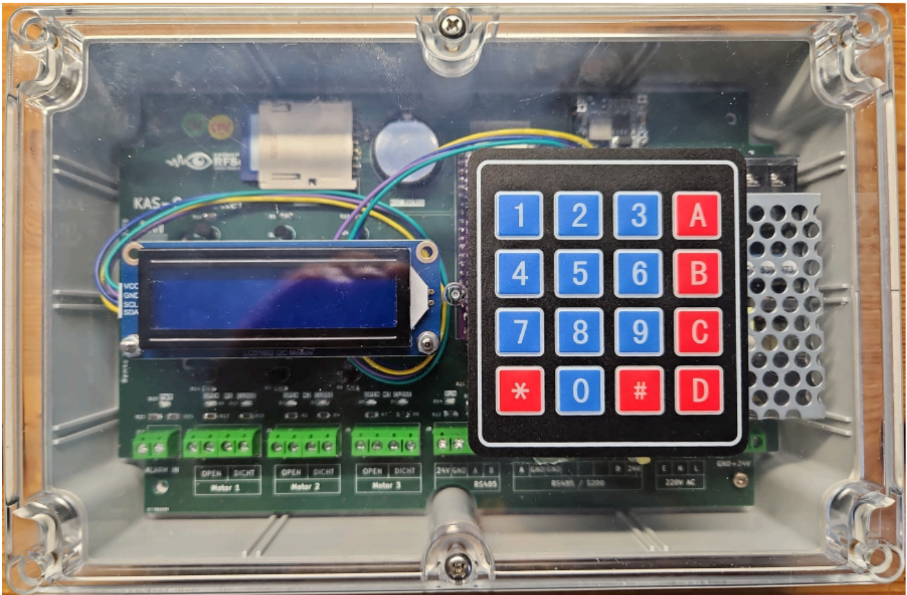
Figuur 4: Kas controller vooraanzicht.
