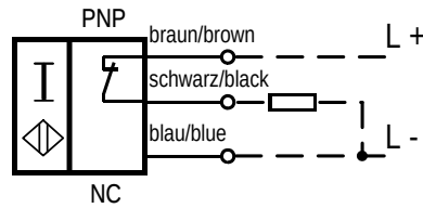
3RG4023-0AA00-PF:
