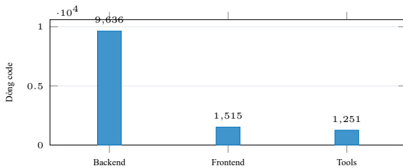
Hình 2: Phân bố dòng code theo module chính.
