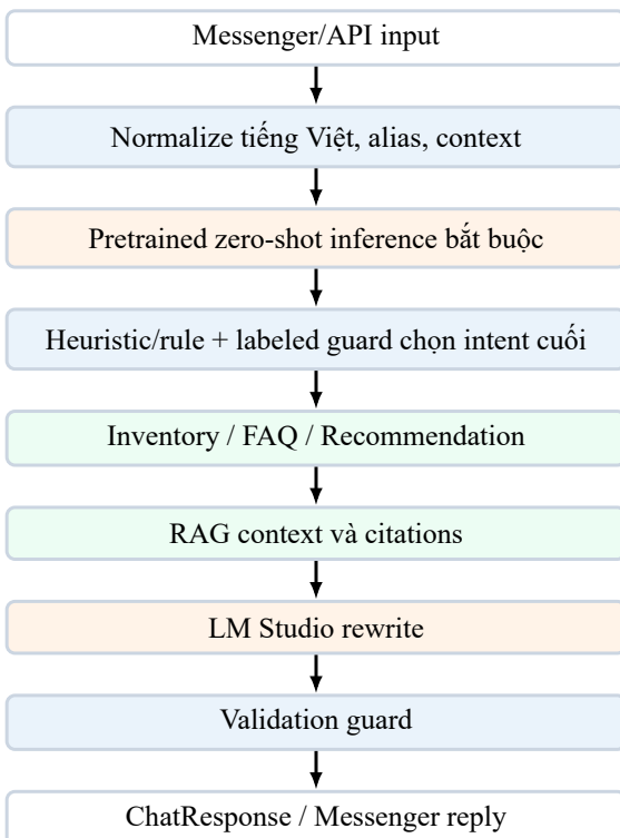
Hình 3: Pipeline xử lý một câu hỏi khách hàng.
