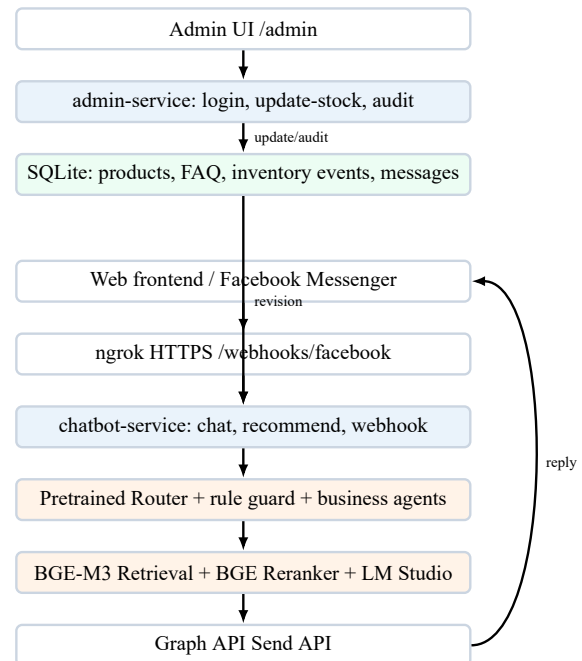
Hình 1: Kiến trúc tổng thể theo luồng dọc.
