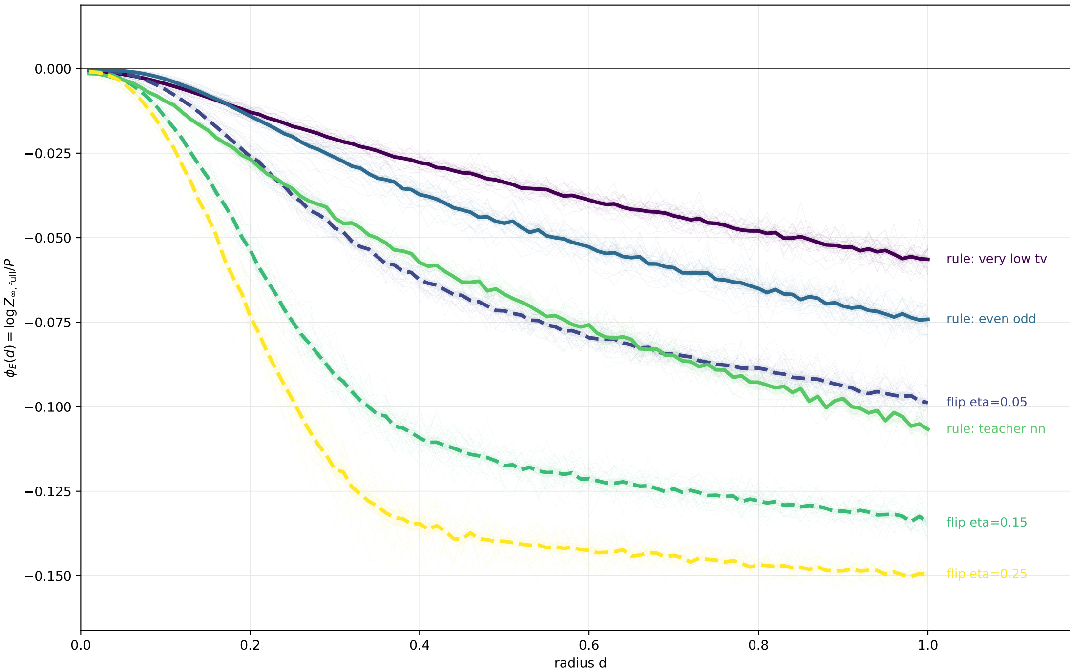
MNIST active rules + eta flips: direct-run raw \phi_E(d)
