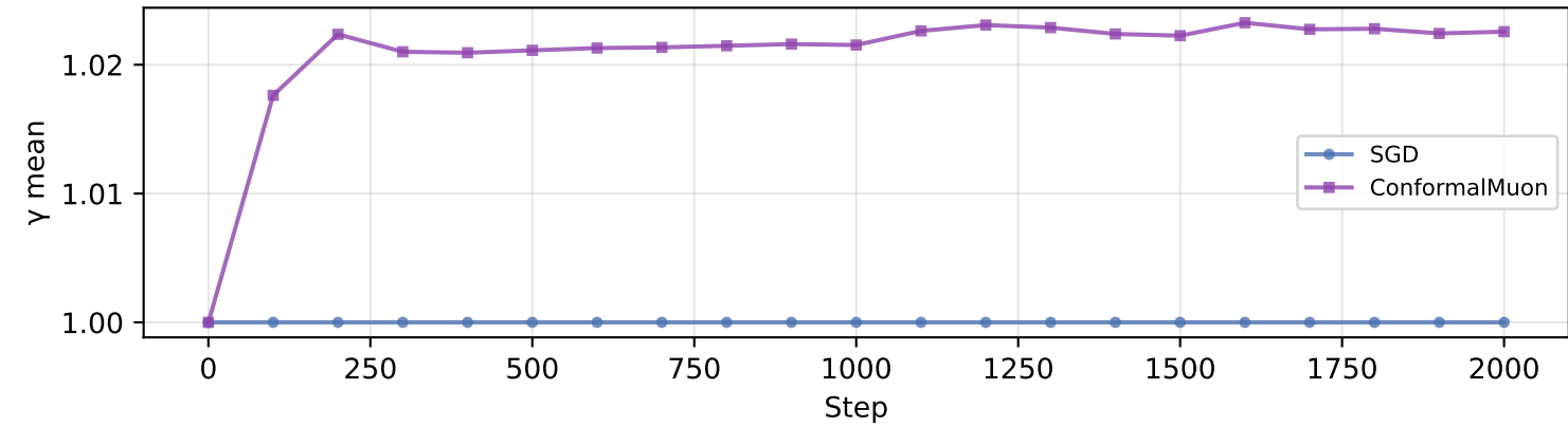
ln_f — \gamma trajectory
