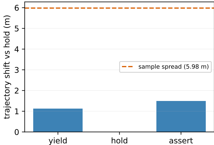
Predicted-response shift
