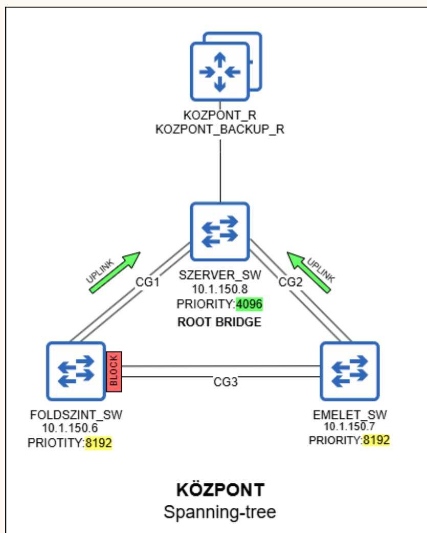
16. ábra: Spanning-tree működése a KÖZPONT telephelyen
