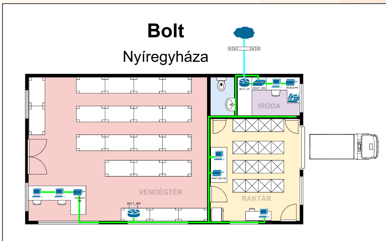
6. ábra BOLT telephely fizikai topológia
