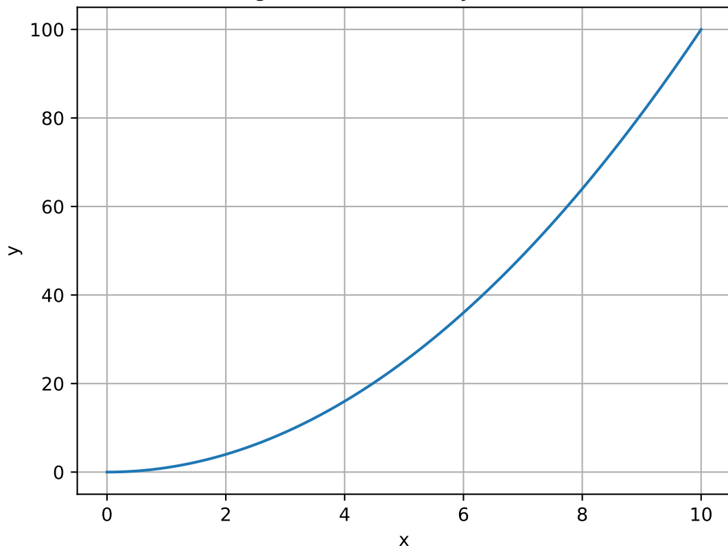
grafico de funcao: y = x^2
