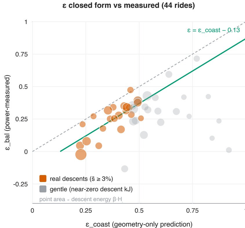
Figura 4. \epsilon_{\text{coast}} apenas-geométrico vs o \epsilon_{\text{bal}} de balanço de descida medido por potência, um ponto por pedalada, área do ponto proporcional à energia de descida \beta \cdot H_- . Em descidas reais ( \bar{s} \geq 3\% , vermelhão) a linha calibrada \epsilon = \epsilon_{\text{coast}} - 0.13 (verde) acompanha a medição; pedaladas suaves (cinza) espalham-se abaixo da linha identidade mas carregam \approx 0 de energia de descida, tornando o erro inofensivo. Vale a ressalva parte-todo acima: \epsilon_{\text{bal}} e \epsilon_{\text{coast}} compartilham seu termo geométrico dominante.
