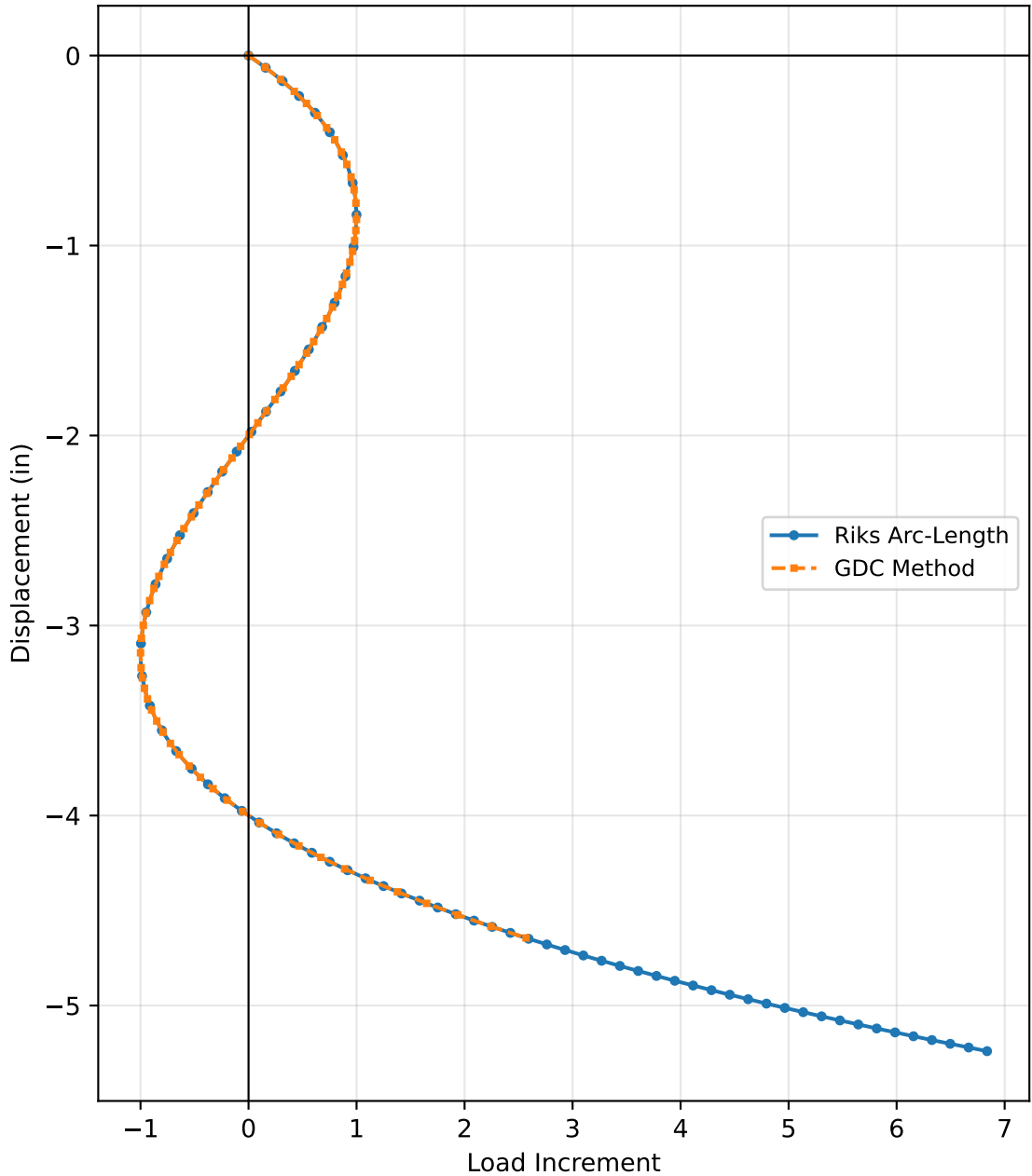
Comparação: Riks vs GDC (Ex 1)
