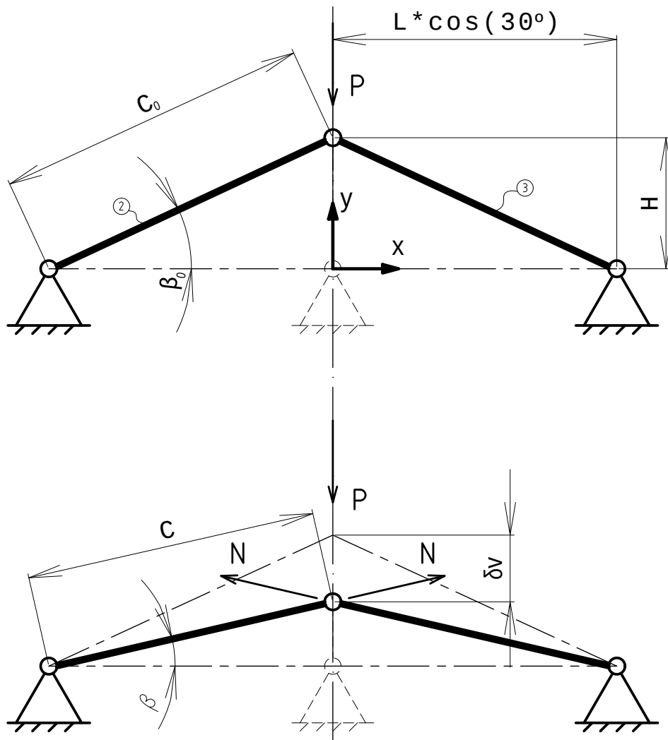
Figura 15: Sistema estrutural do Trabalho Prático 08 – Vista lateral
