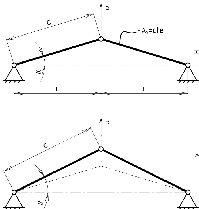
Figura 16: Sistema estrutural do Trabalho Prático 09.
