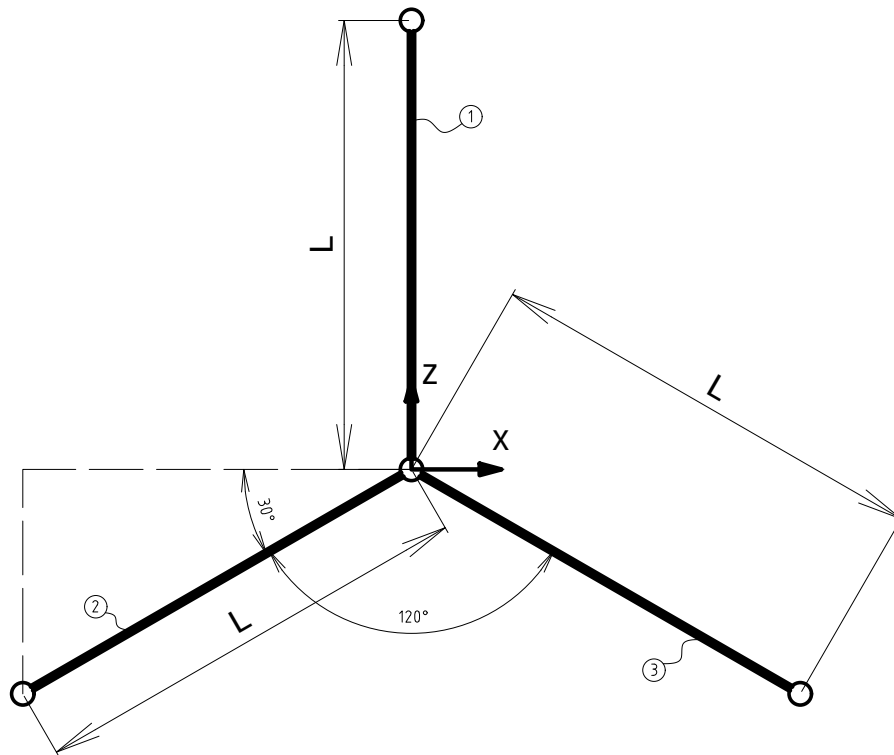
Figura 14: Sistema estrutural do Trabalho Prático 08 – Vista superior
