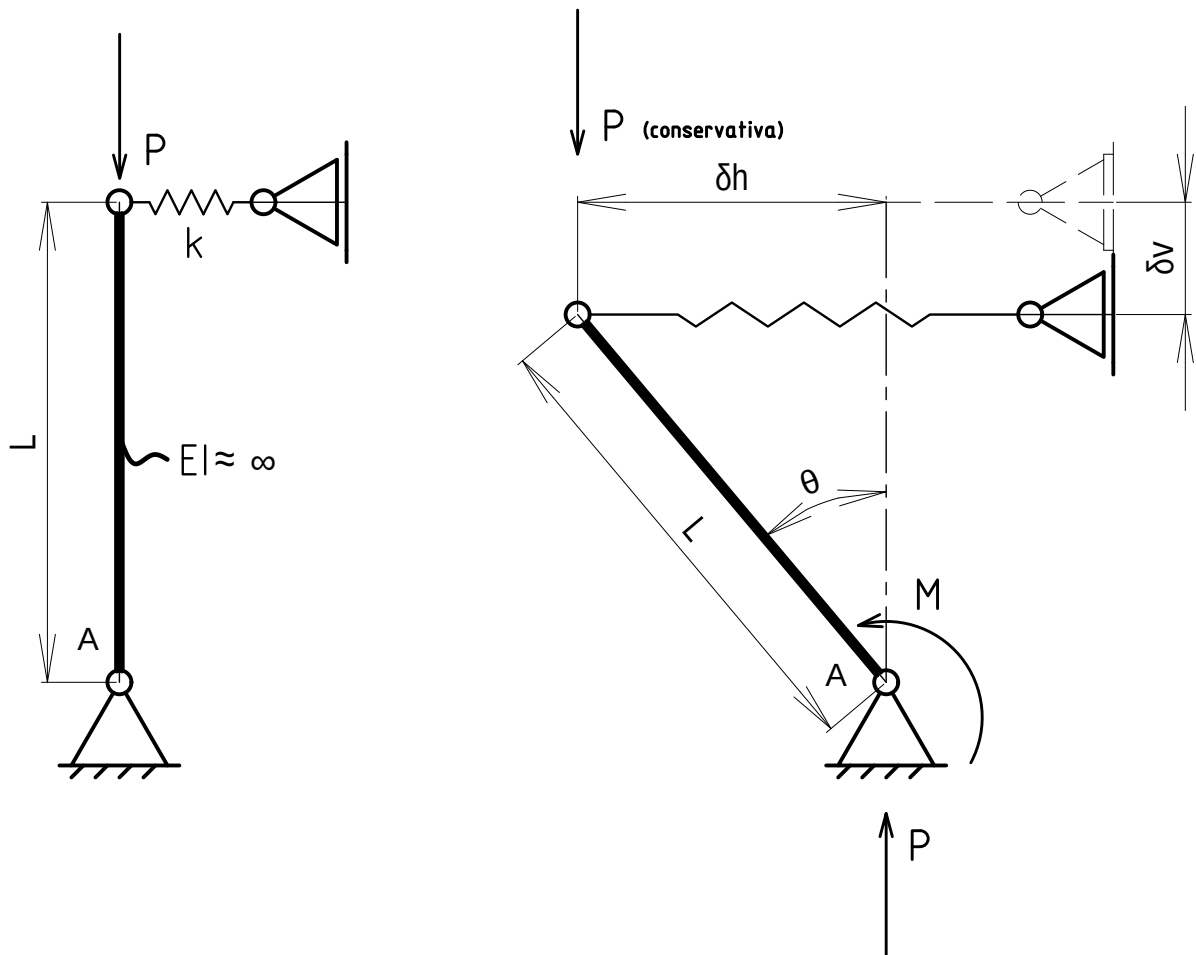
Figura 3: Sistema estrutural do Trabalho Prático 02.
