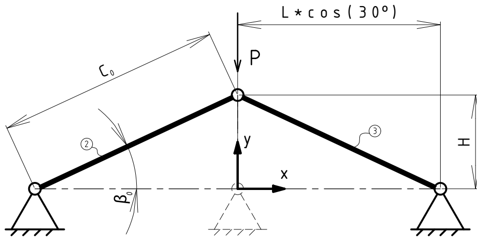
Figura 9: Sistema estrutural do Trabalho Prático 08 – Vista lateral
