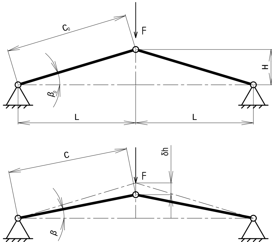
Figura 7: Sistema estrutural do Trabalho Prático 05.
