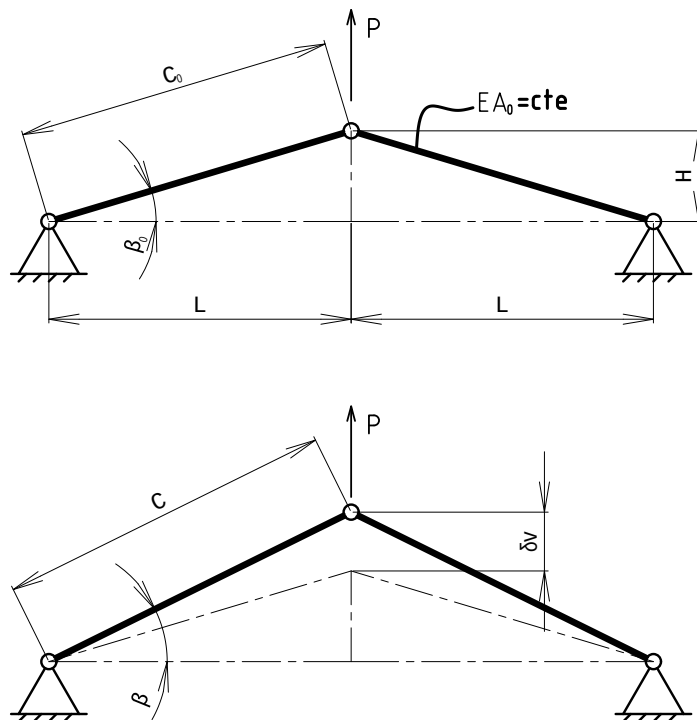
Figura 10: Sistema estrutural do Trabalho Prático 09.
