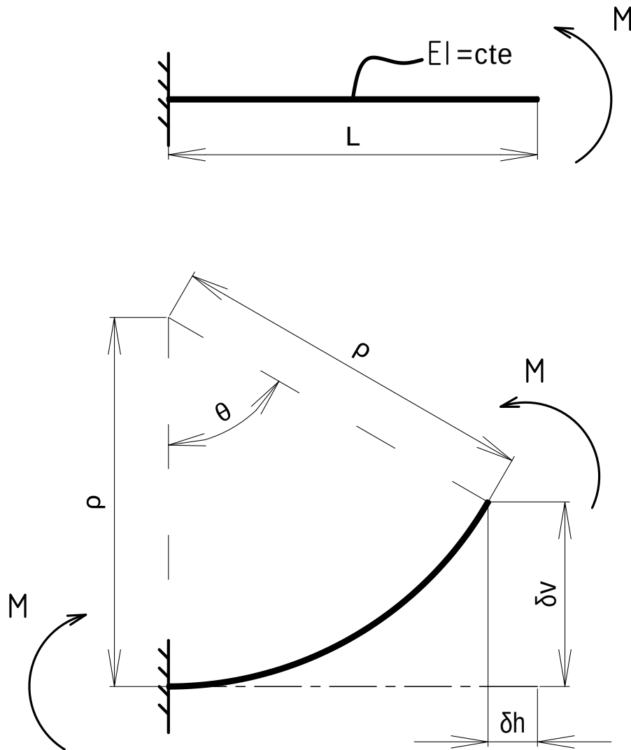
Figura 6: Sistema estrutural do Trabalho Prático 04.
