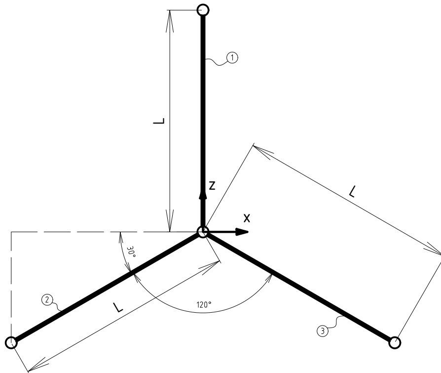
Figura 8: Sistema estrutural do Trabalho Prático 08 – Vista superior
