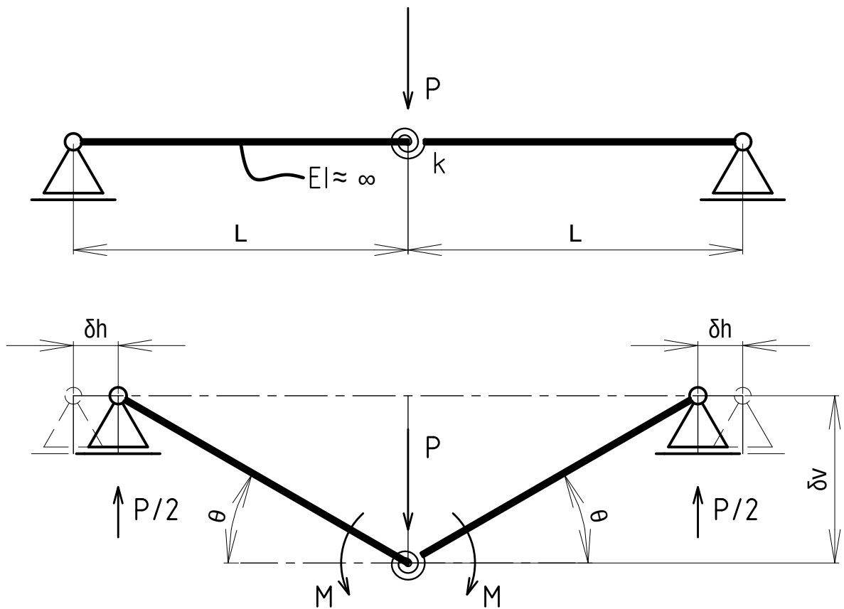
Figura 5: Sistema estrutural do Trabalho Prático 03.
