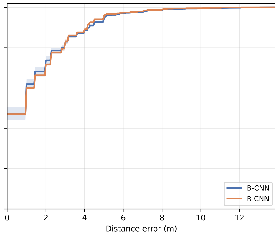
(b) B-CNN vs R-CNN (Fusion)
