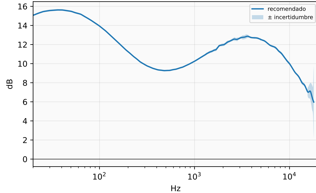
Guitarra — detalle
