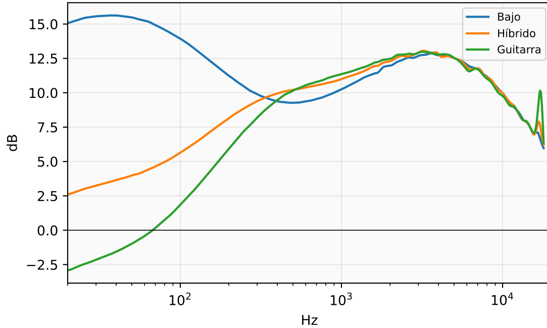
Híbrido — detalle
