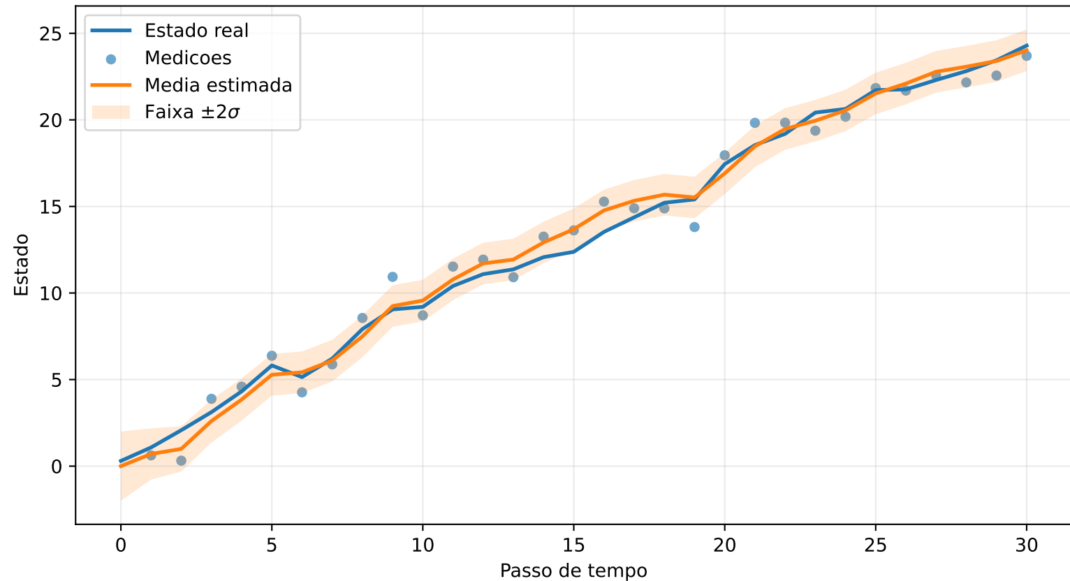
Questao 10 - Filtro de Bayes 1D (RMSE = 0.559)
