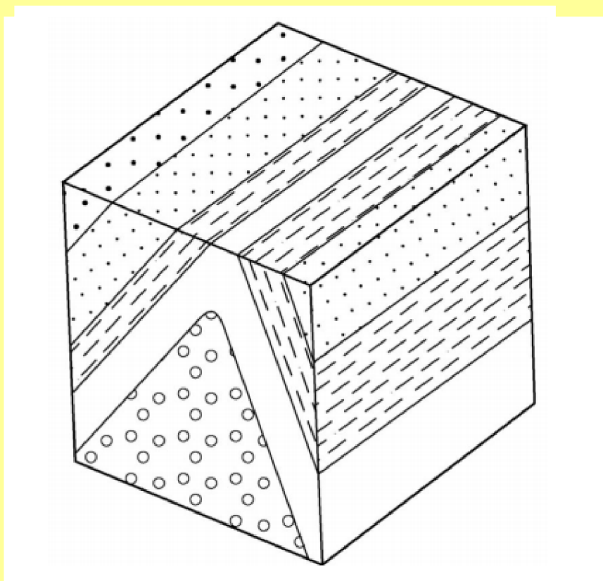
ANTICLINAL
