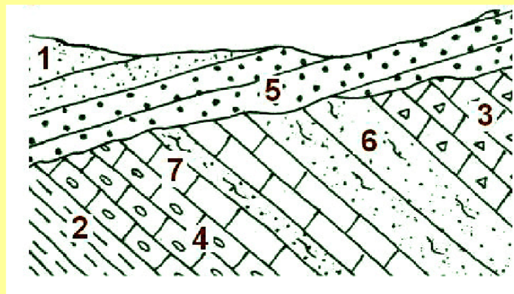
Basculament
