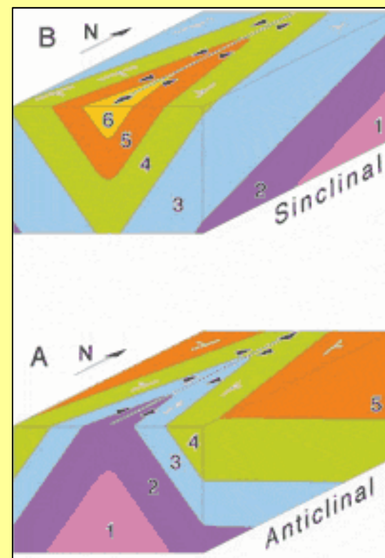
Plec anticlinal o sinclinal
