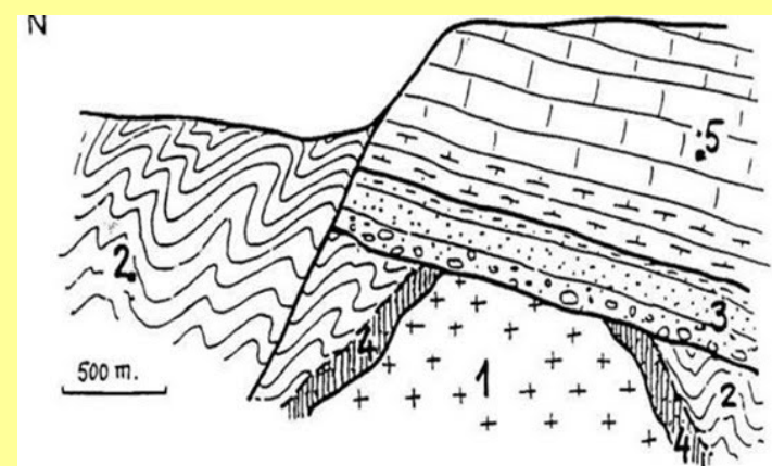
Intrusió
