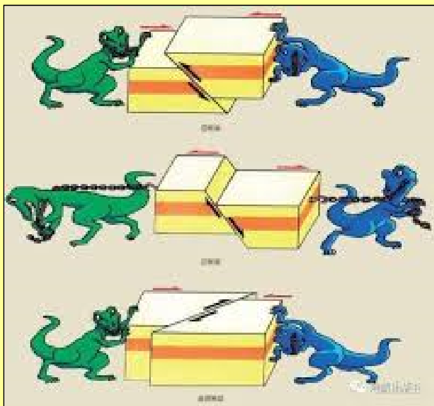
Falla normal, inversa o transformant
