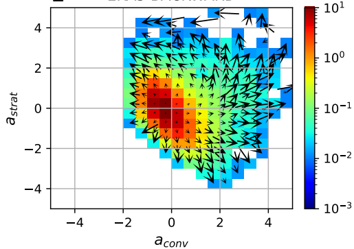
E ERA5 BACKWARD
