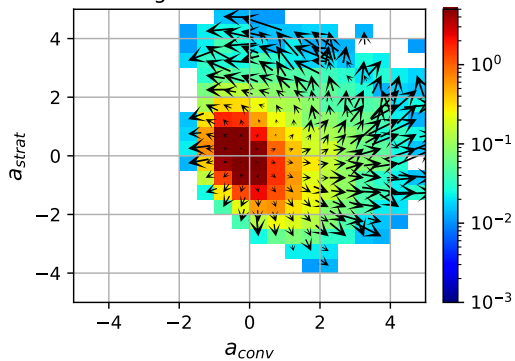
B gSAM BACKWARD
