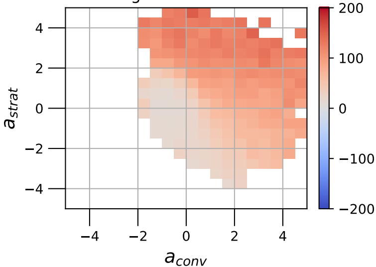
gSAM LW CRE
