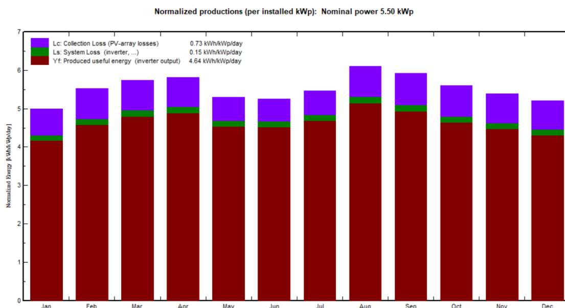
Figura 7.1 — Estimativa de geração de energia mensal do SFCR.
