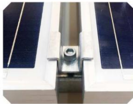
(b) Grampo intermediário.
