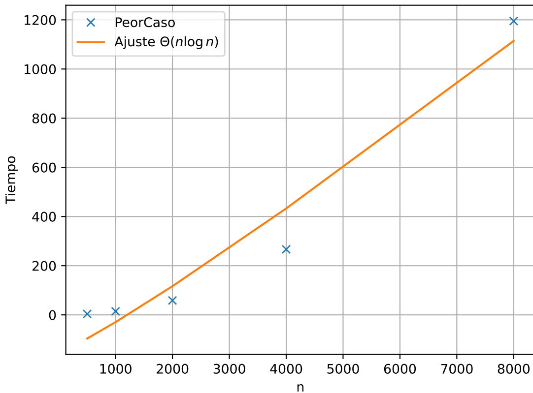
Peor caso \sim \Theta(n \log n)
