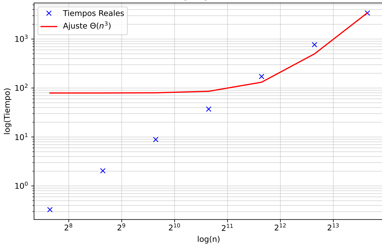
Peor Caso: Escala Log-Log (Verificación de Potencia)
