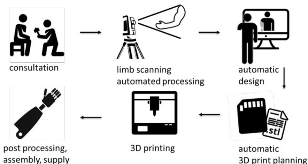
Figura 5.1 — Fluxo geral de produção personalizada de próteses a partir de digitalização, CAD adaptativo e fabrico aditivo.
