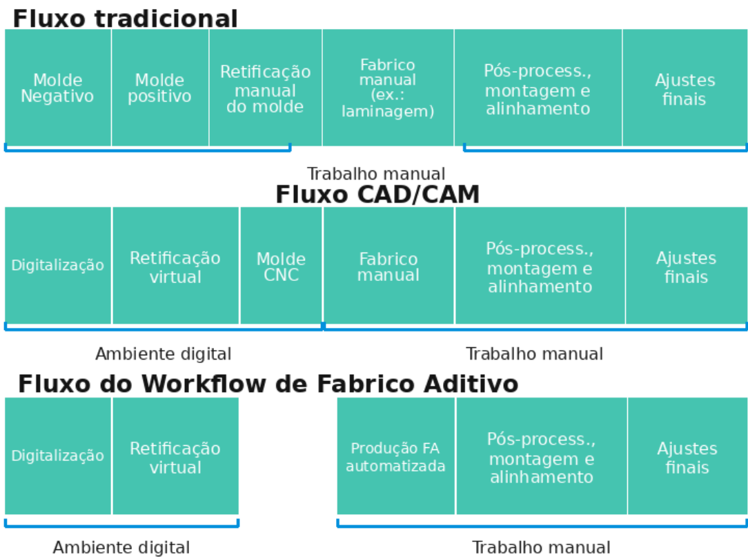
Figura 2.3 — Fluxo digital entre aquisição, CAD/CAM e fabricação aditiva em próteses e ortóteses.
