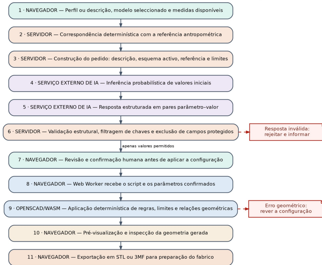
Figura 5.4 — Sequência de dados e decisões desde o perfil ou descrição até à sugestão, confirmação, geração determinística e exportação.
