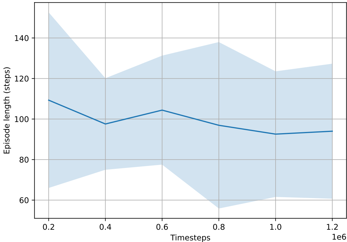
Longitud de episodio (Evaluación): media \pm std
