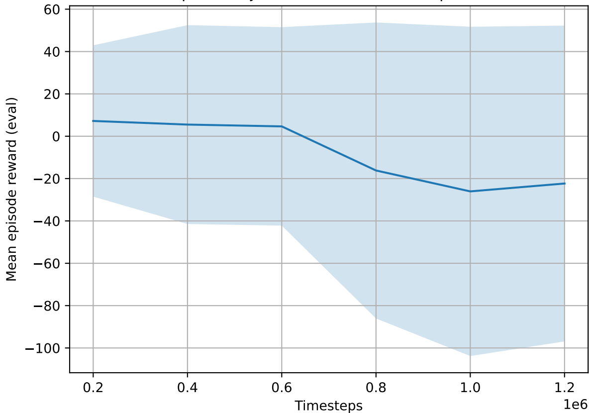
Curva de aprendizaje (Evaluación): reward promedio \pm std
