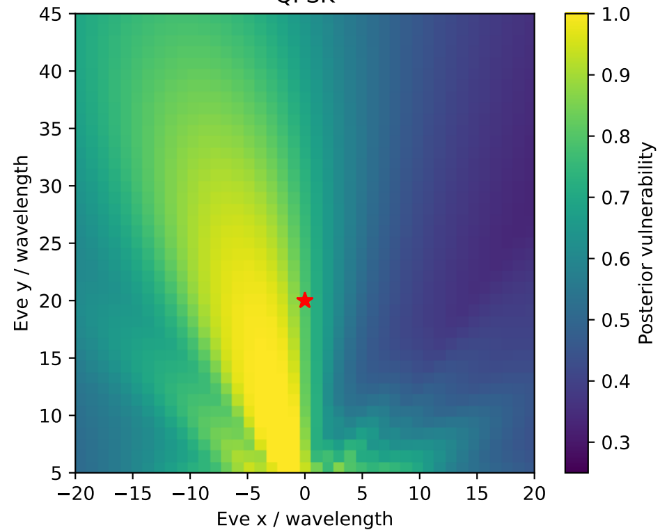
QPSK
