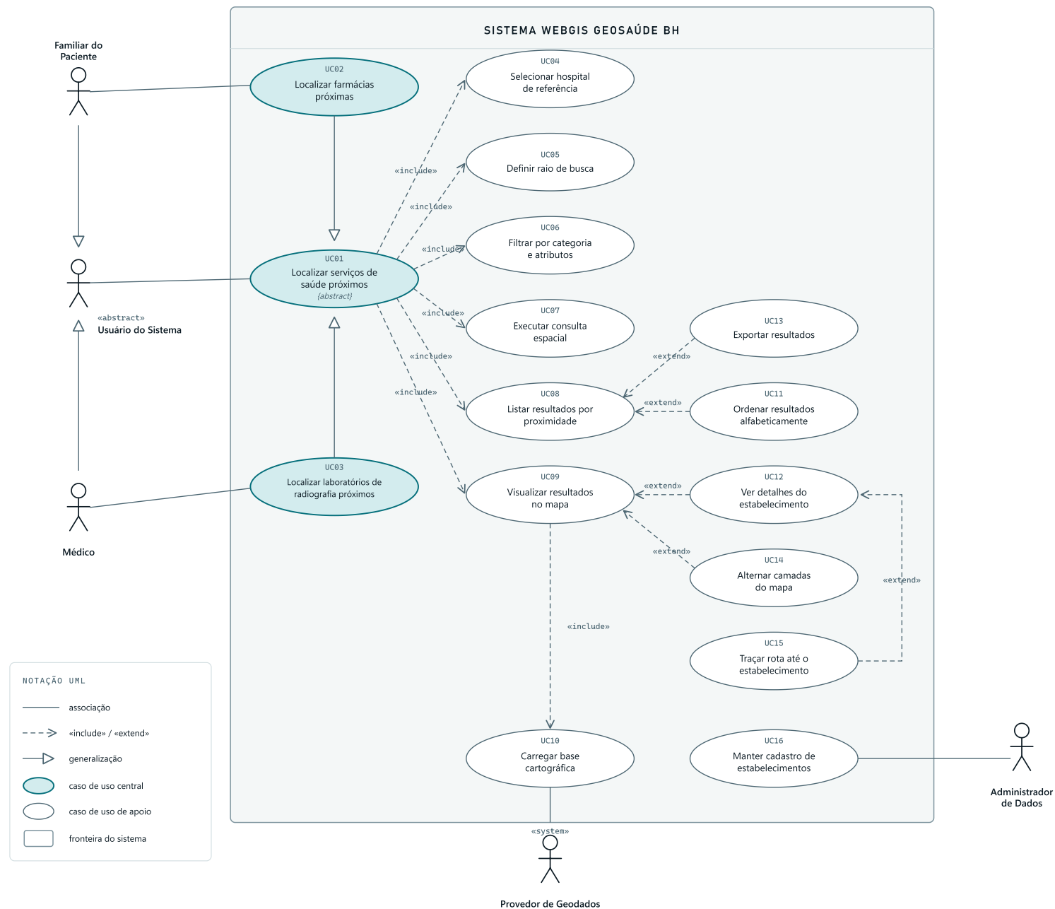
Fig. 1 – Diagrama de casos de uso · UML 2.5 · GeoSaúde BH
