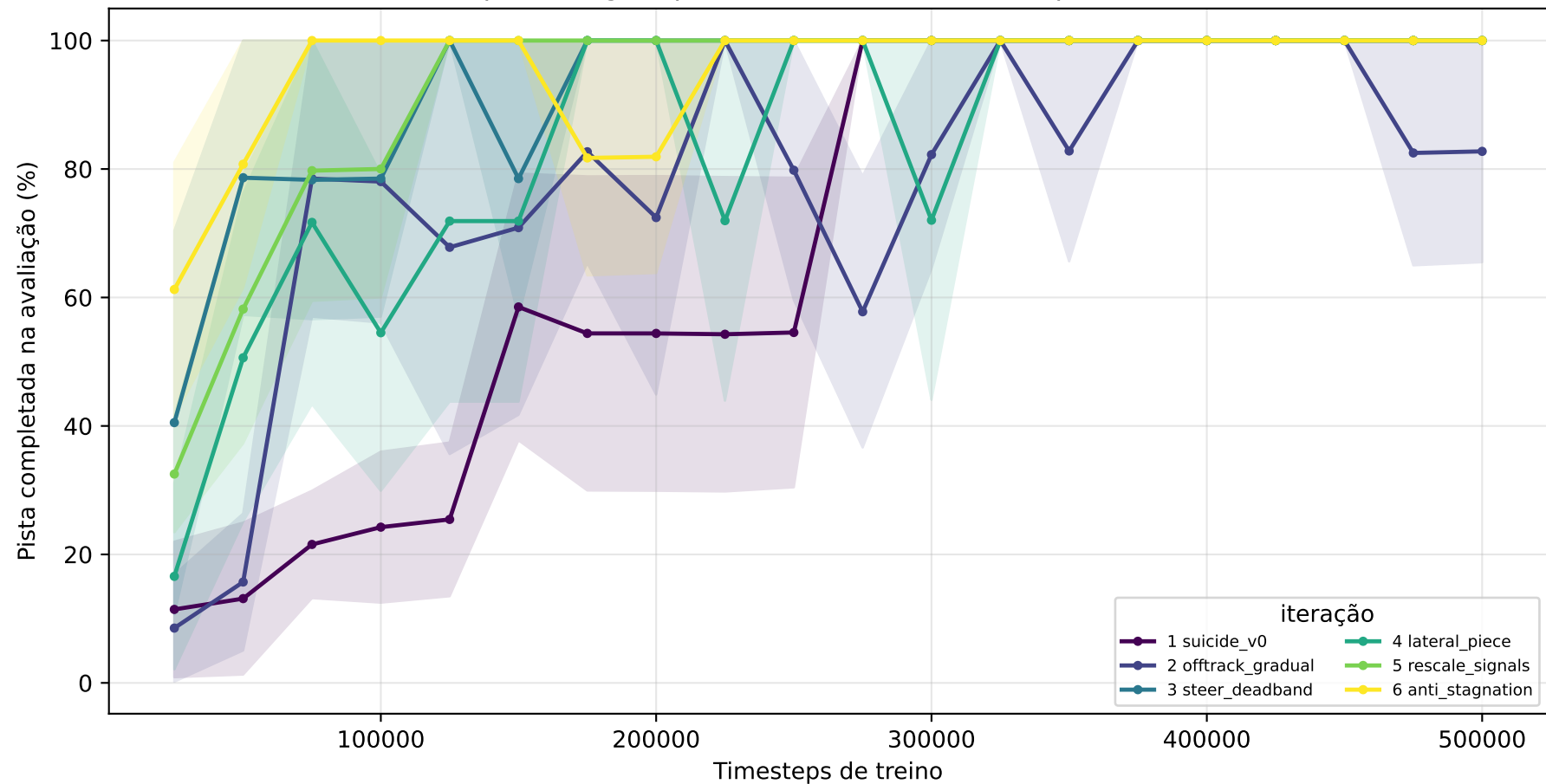
Curvas de aprendizagem por iteração (média \pm erro-padrão sobre seeds)
