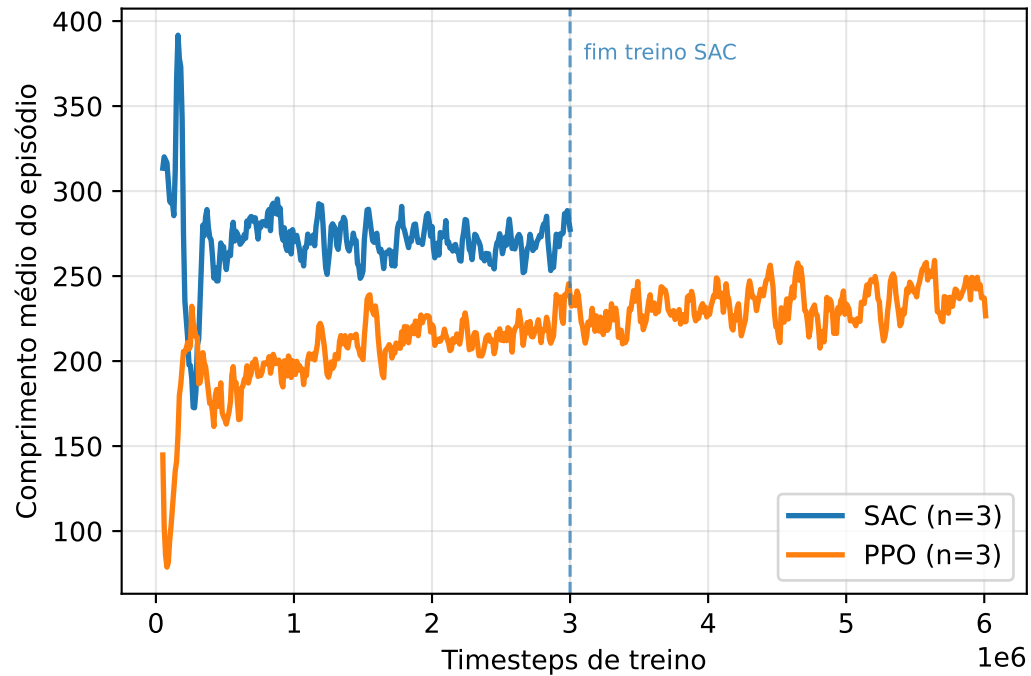
Estabilidade do agente
