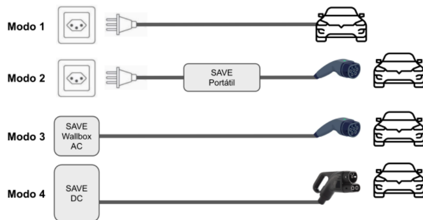
Figura 1: Modos de recarga de acordo com a norma ABNT NBR IEC 61851-1
