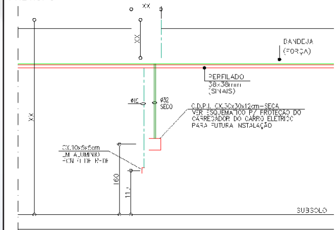
CARREGADOR P/ CARRO ELÉTRICO VISTA PARA PONTOS DA INSTALAÇÃO DO CARREGADOR VEICULAR PREVISÃO
