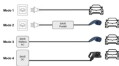
Figura 2: Esquema dos modos de carregamento (NBR IEC 61851-1)
