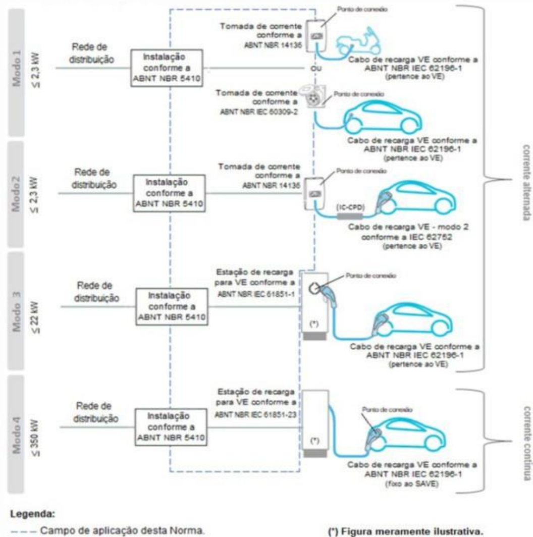
Figura A.5 – Campo de aplicação desta Norma ao integrar um SAVE à instalação elétrica fixa
