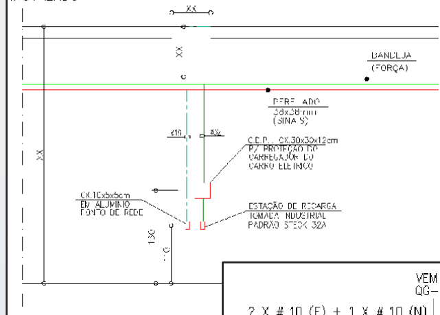
CARREGADOR P/ CARRO ELÉTRICO VISTA PARA PONTOS DA INSTALAÇÃO DO CARREGADOR VEICULAR INSTALADO
