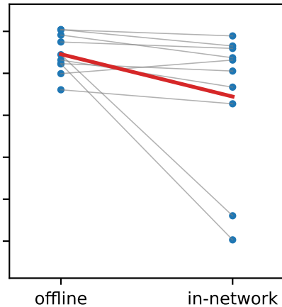
CatBoost
