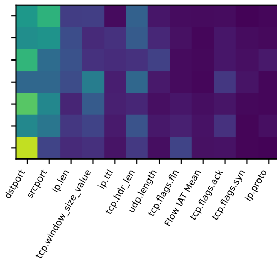
CatBoost
