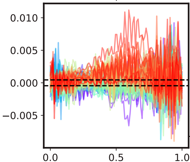
Eq 6
