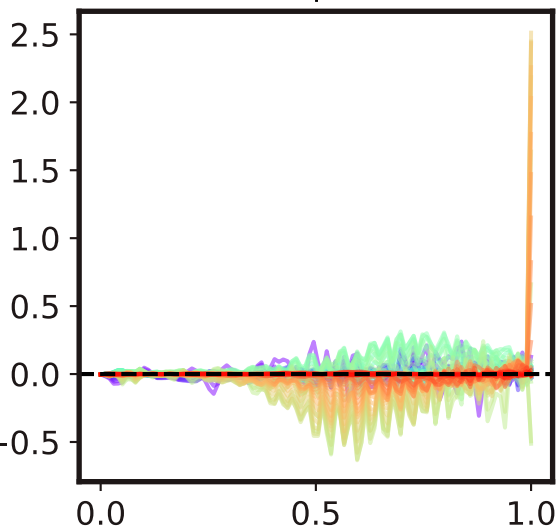
Eq 7
