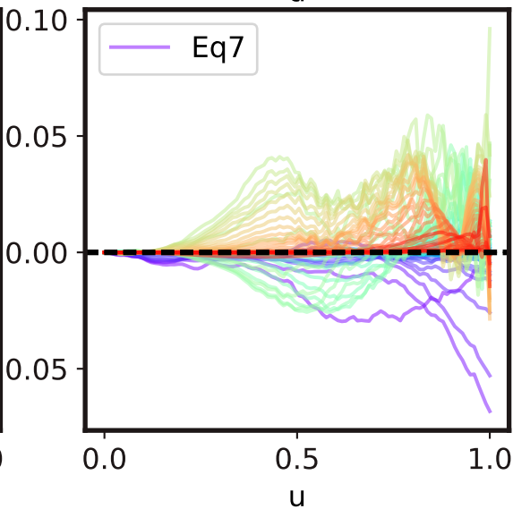
Eq 7
