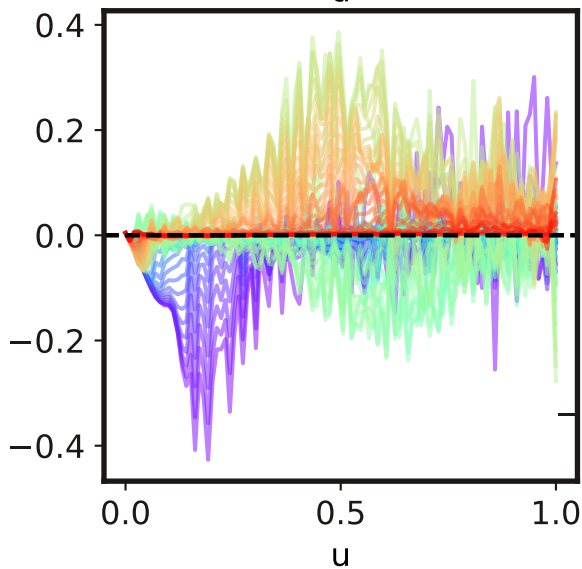
Eq 6
