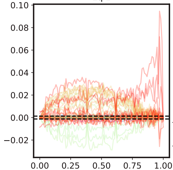
Eq 1
