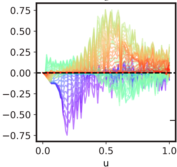
Eq 6
