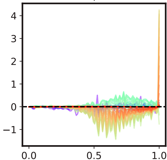
Eq 7
