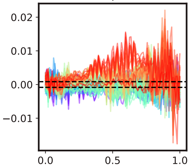
Eq 6
