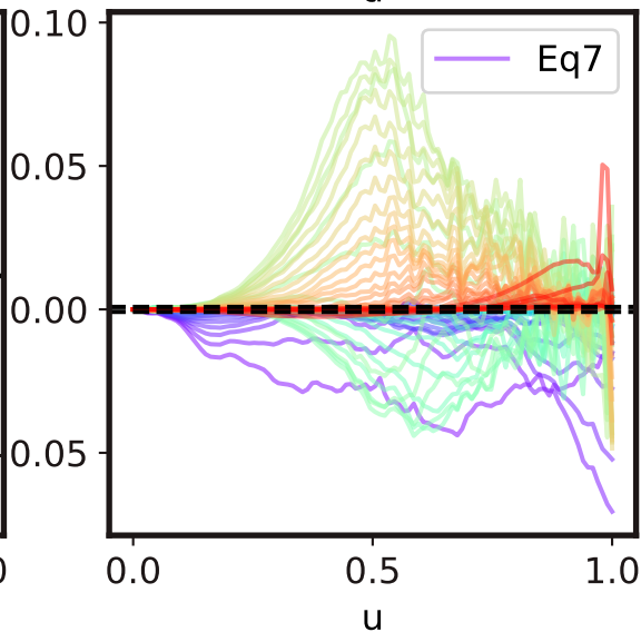
Eq 7
