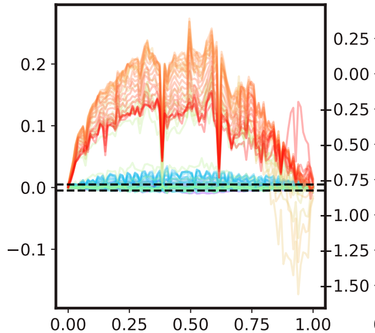
Eq 1
