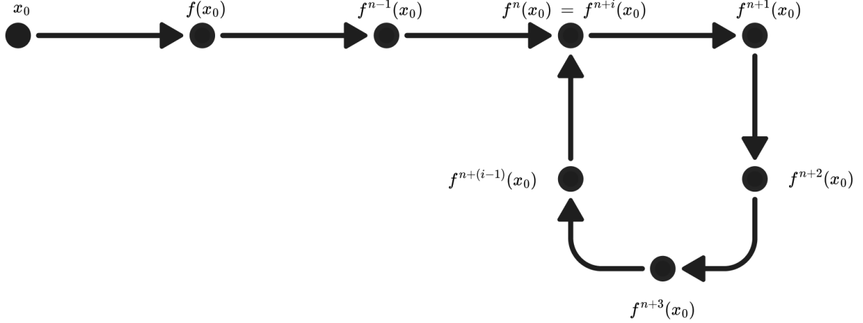
Figura 2.1: Ponto eventualmente periódico.
