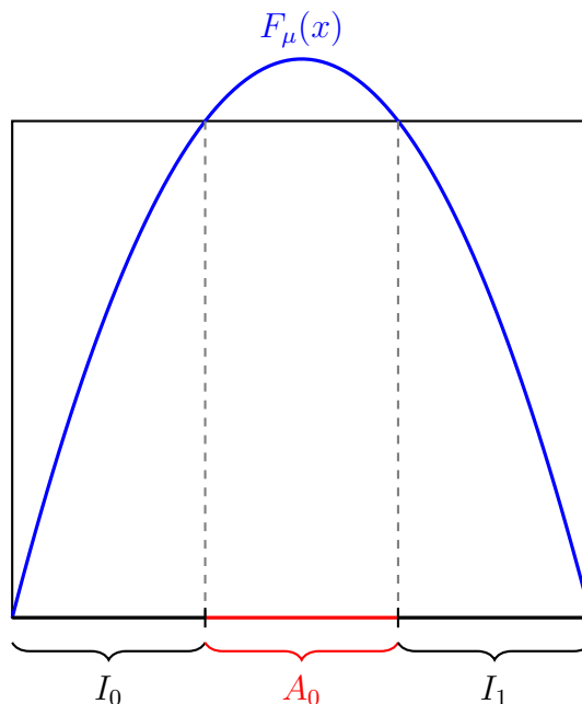
Figura 4.4: Ilustração dos intervalos I_0 , A_0 e I_1
