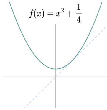
Figura 3.2: Análise da parábola com parâmetro \mu = \frac{1}{4}
