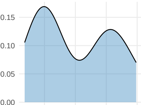
limma-CLR
