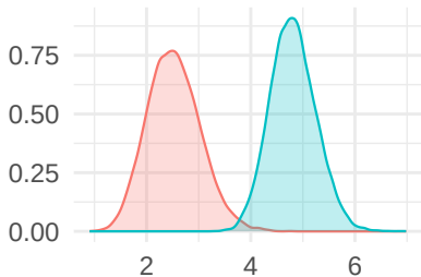
4: monoacetiladas / diacetiladas
