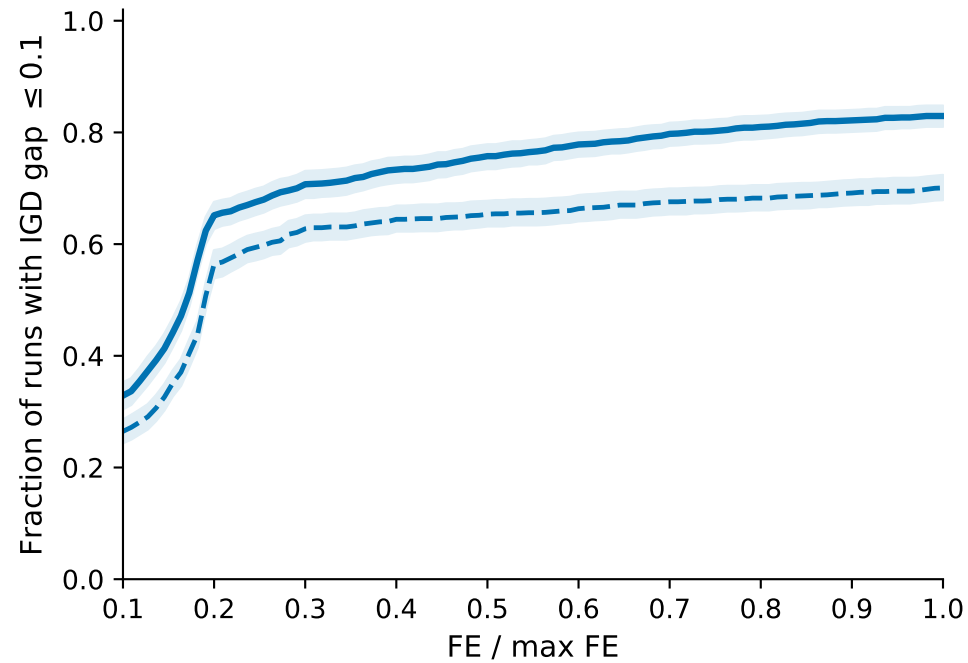
IVF/SPEA2
