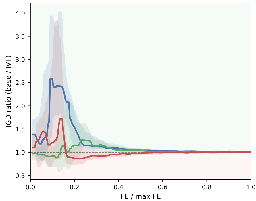
ZDT4 ( M = 2 )
