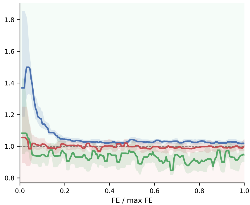
DTLZ5 ( M = 3 )
