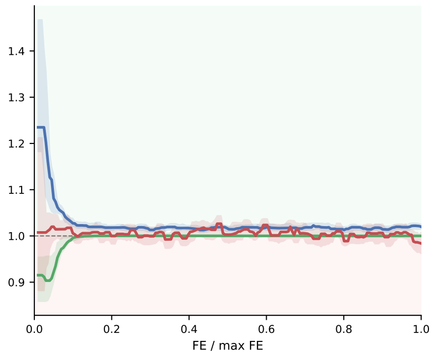
DTLZ5 ( M = 3 )
