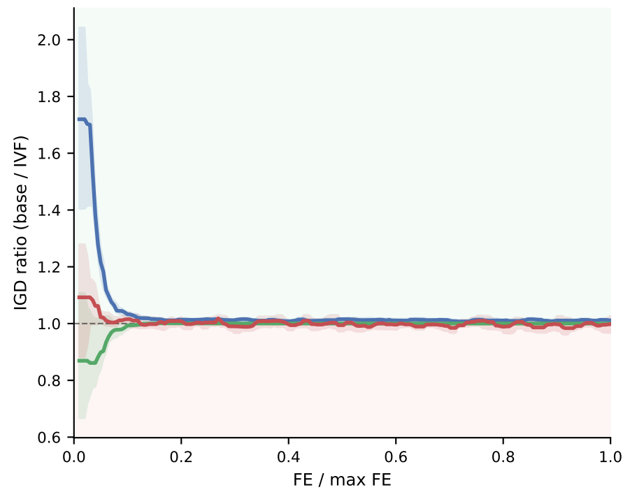
ZDT4 ( M = 2 )
