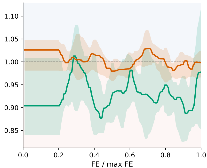
DTLZ5 ( M = 3 )
