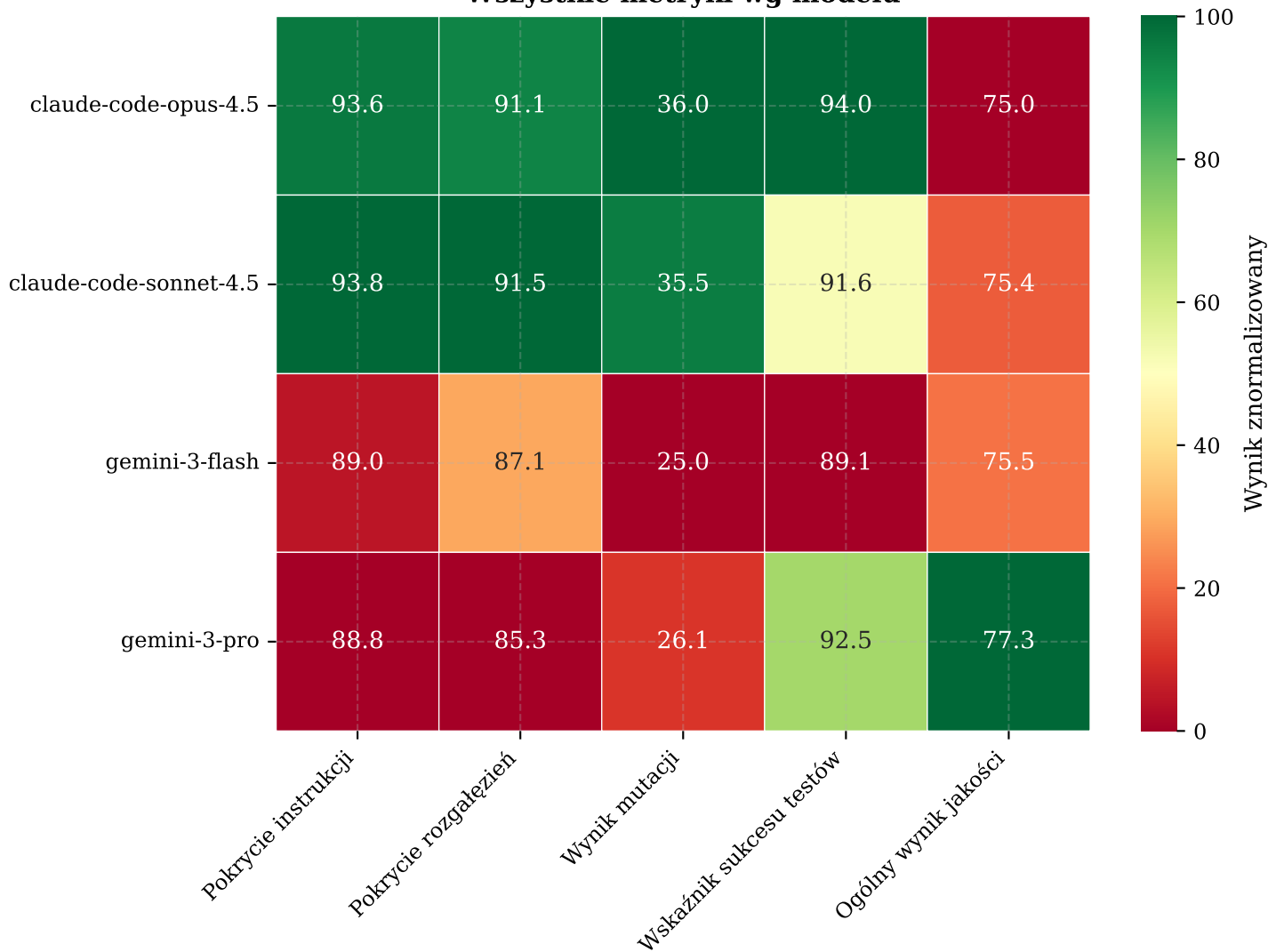
Wszystkie metryki wg modelu
